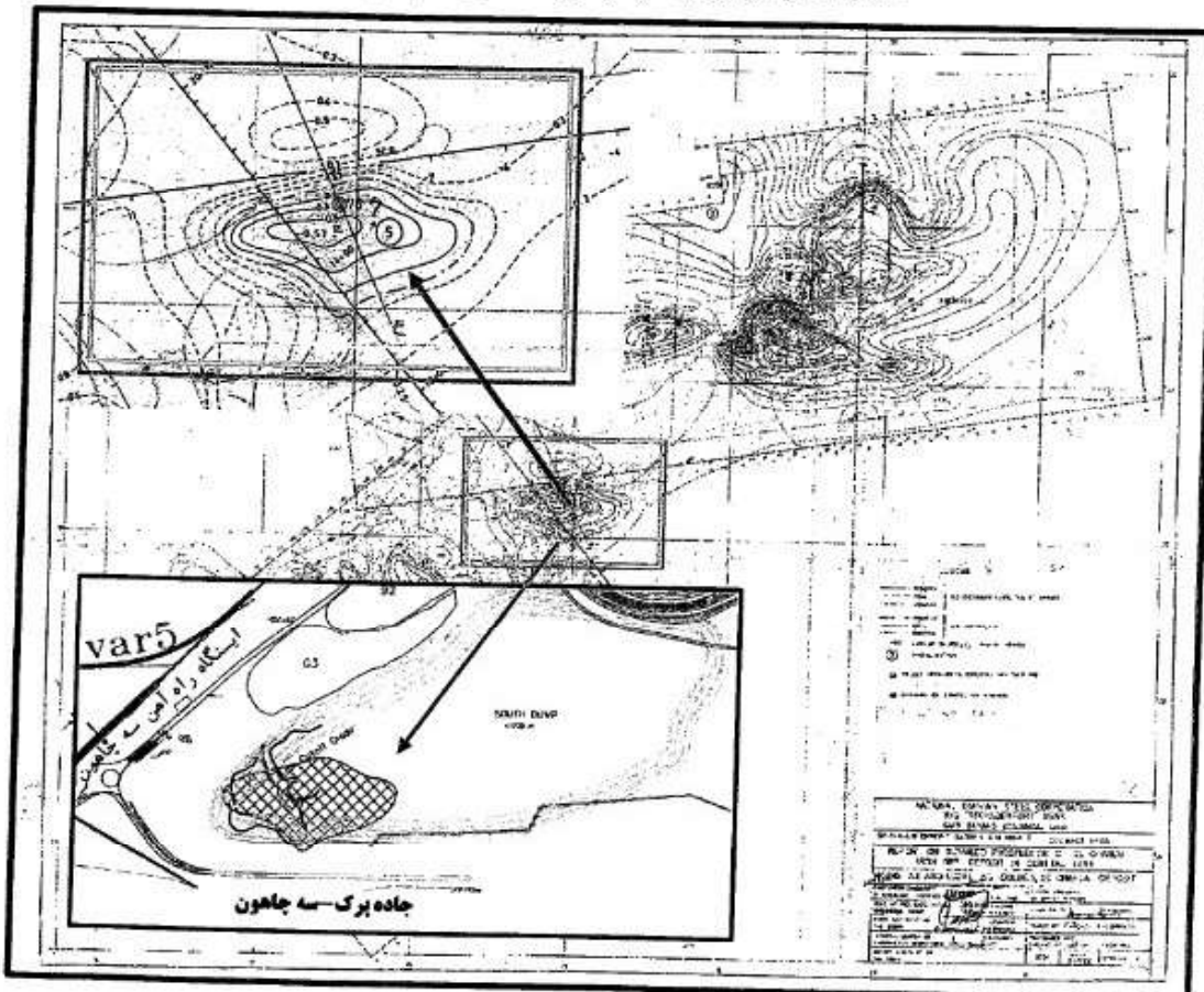
شکل ۴: آنومالی فرعی ۵ از آنومالی ۱۱ معدن سه چاهون
