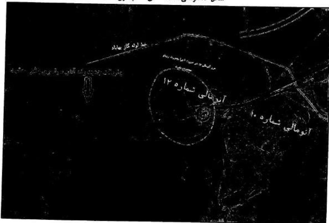
شکل ۶: آنومالی ۱۲ A معدن سه چاهون
